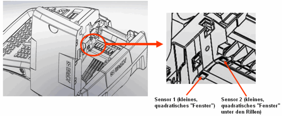
Abbildung14 • Lage der Sensoren
